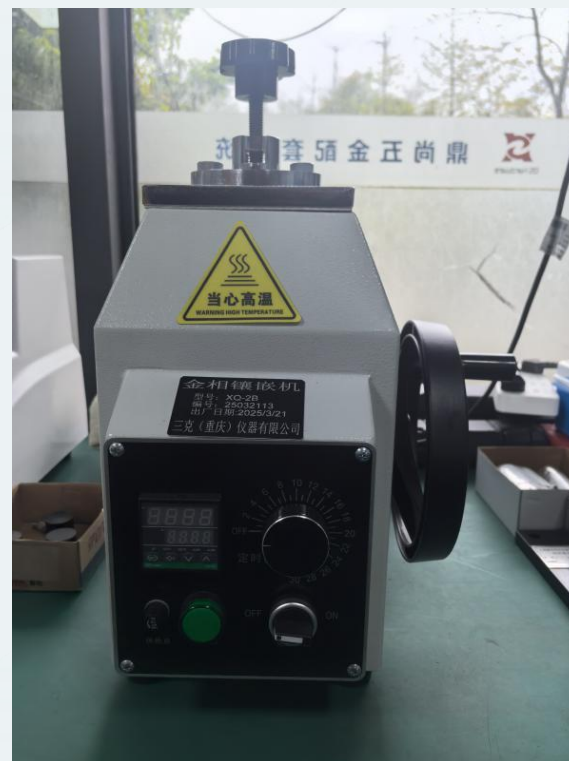
金相分析仪
